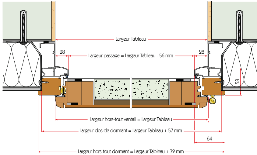
COUPE HORIZONTALE
