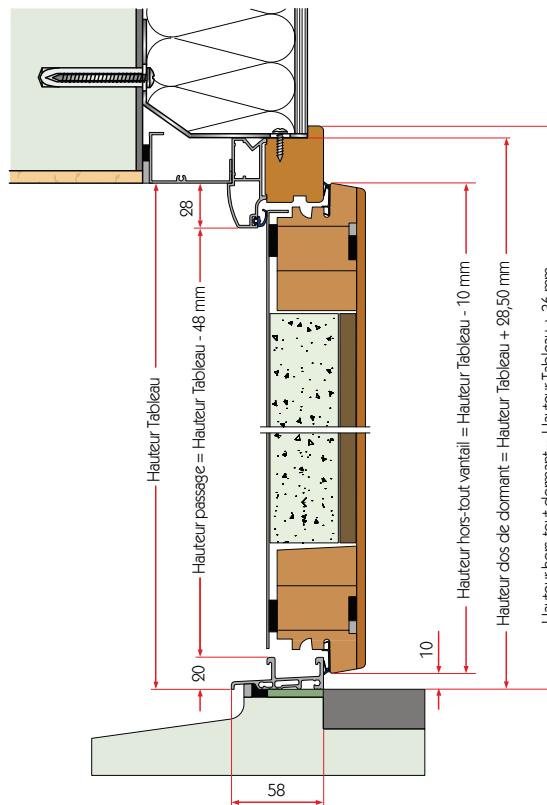
COUPE VERTICALE
