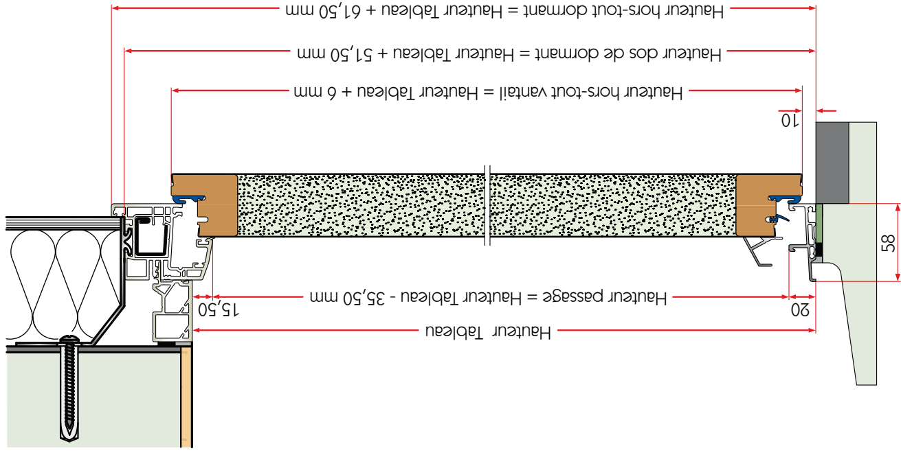
COUPE VERTICALE AVEC DORMANT PVC
