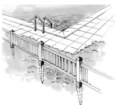
Fixation de clôtures à enfonceur dans le sol
