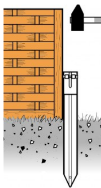
Fixation de palissades à enfonceur dans le sol
