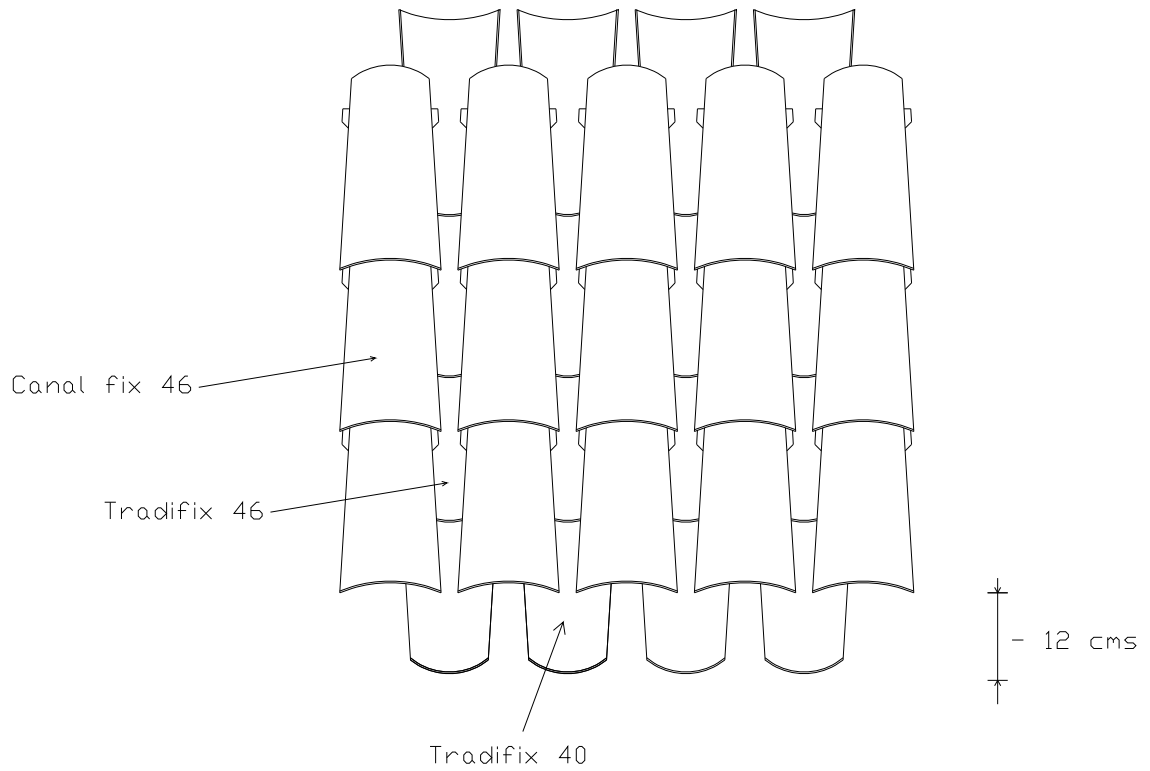
Figure 9 – Débord de toit -12 cm
