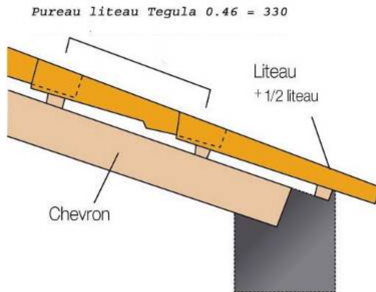
Figure 5 - Pose sur liteau
