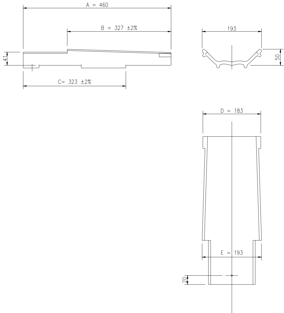
Figure 1 – Tuile de courant MULTIFIX 0,46
