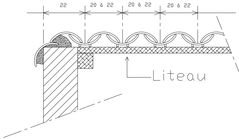
Figure 12 – Rive de tête sans dépassement de mur
